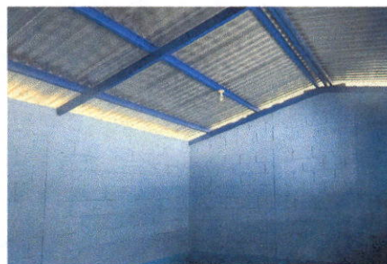
Foto 2: Sustitución de estructura de soporte de madera por metal y sustitución de lámina
